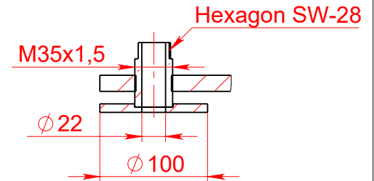
SECTION B-B SCALE 1 : 5
